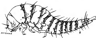
Fig. 186. Hydroscapha natans Lec.
